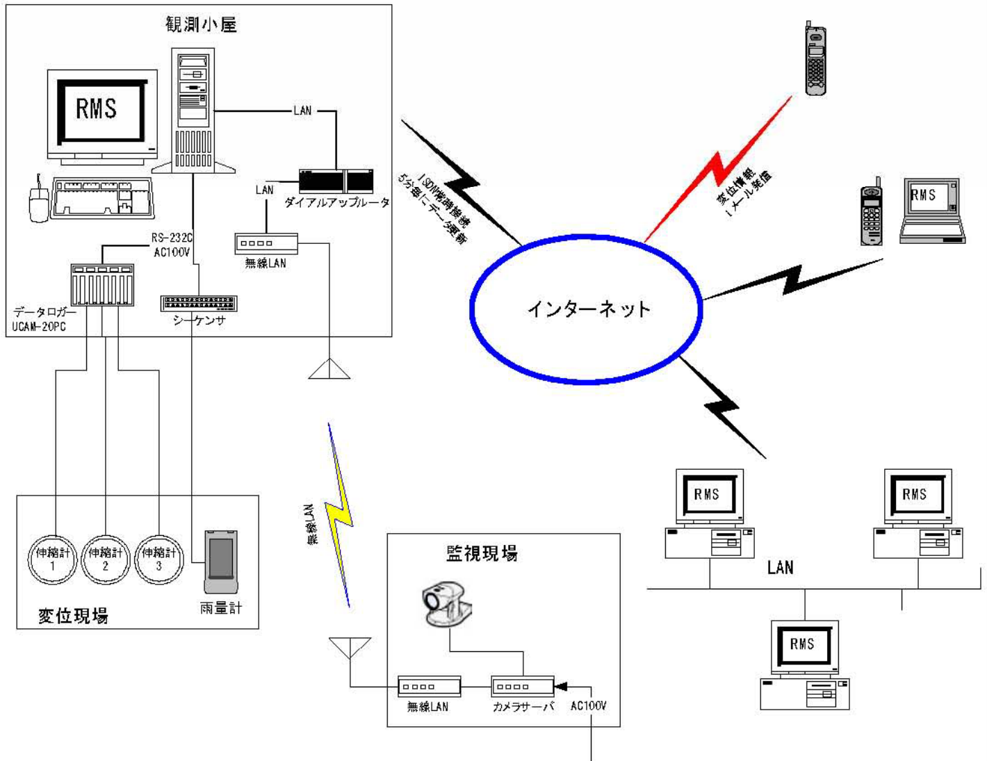
RMS監視 システム図
